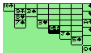
Klondike solitaire
