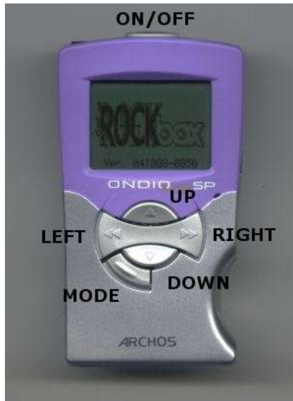
Ondio 128
